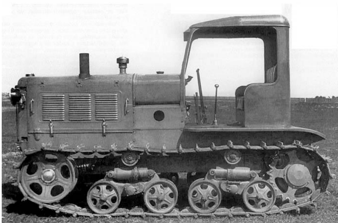
Трактор СТЗ-НАТИ
