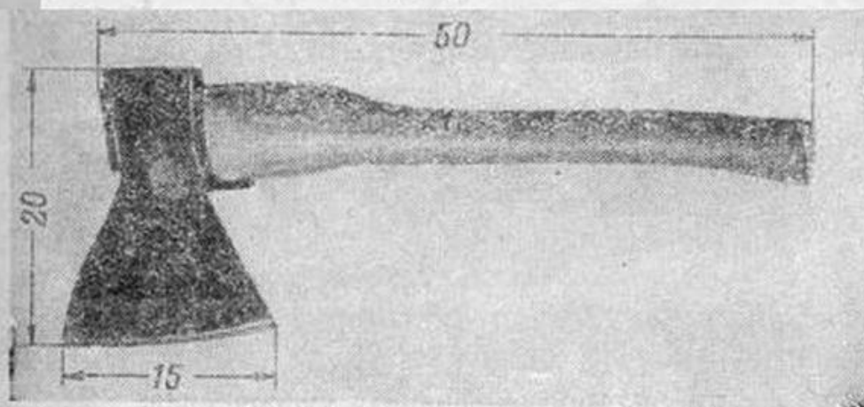
Рис. 6. Топор плотничный
