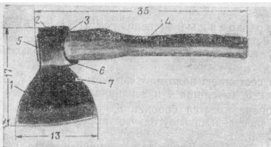
Рис. 5. Топор военный (специальный): 1 — лезвие; 2 — обух; 3 — всад; 4 — топоричце; 5 — заклинок; 6 — борода; 7 — вырез
